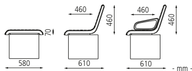
Mauerauflage PORT mit und ohne Rückenlehne, Breite 580 mm und 1820 mm, mit Robinienholzbelattung
