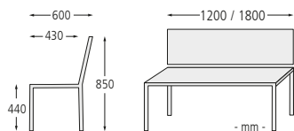
▲ Sitzbank MONZA, Breite 1800 mm, in RAL 6005 moosgrün
