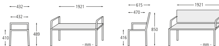
Bank-Tisch-Kombination TORRE bestehend aus Sitzbank mit und ohne Rückenlehne und einem Tisch, in RAL 6005 moosgrün
