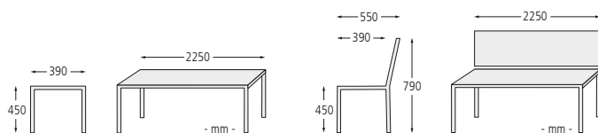
▲ Sitzbank VEGA ohne Rückenlehne, Stahlteile in RAL 7021 schwarzgrau, Beton beschichtet in Farbe graphit
