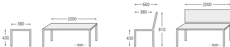
Bank-Tisch-Kombination VENEDIG, mit Escheholzbelattung, bestehend aus einem Tisch und Sitzbank ohne und mit Rückenlehne
