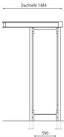
Seitenansicht
