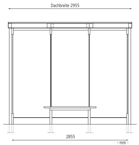
Frontansicht
