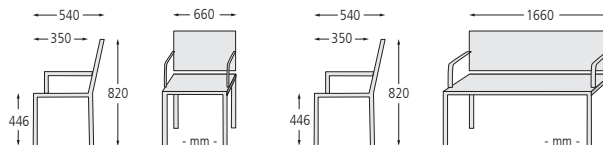
Sitz- und Sitzbank BASIC, Stahlteile in RAL 7016 anthrazitgrau (Abfallbehälter BASIC Online-Angebot)
