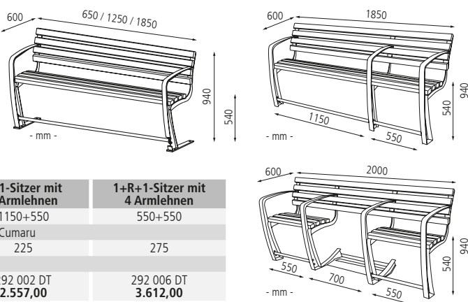
Sitzbank SENIOR, 2-Sitzer mit Armlehnen
