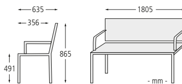
Sitzbank DIVA SOLO-SENIOR mit Robinienholzbelattung, Stahlteile in DB 703 eisenglimmer
