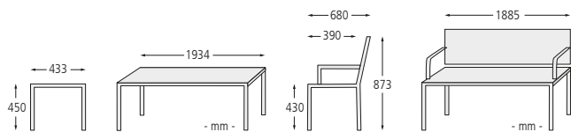
Sitzbank GLURNS ohne Rückenlehne und Tisch GLURNS, in RAL 3000 feuerrot
