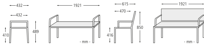
Bank-Tisch-Kombination TORRE bestehend aus Sitzbank mit und ohne Rückenlehne und einem Tisch, in RAL 6005 moosgrün
