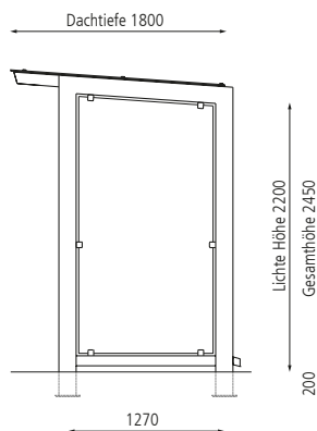
Seitenansicht
