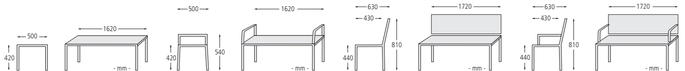
Sitzbank FLOWING mit Rückenlehne und Armlehnen
