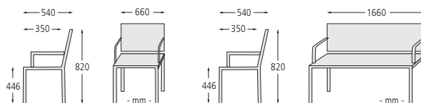
Sitz- und Sitzbank BASIC, Stahlteile in RAL 7016 anthrazitgrau (Abfallbehälter BASIC Online-Angebot)
