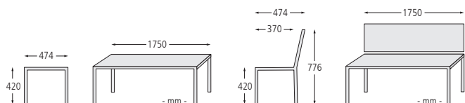
Sitzbank FOLA mit Rückenlehne, Stahlteile in eisenglimmergrau
