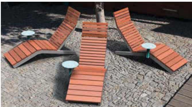
Liegebänke RIVAGE mit Ablagetisch, mit Jatobaholzbelattung, zum freien Aufstellen, Stahlteile in DB 703 eisenglimmer (Ablagetisch in Sonderfarbe auf Anfrage)
