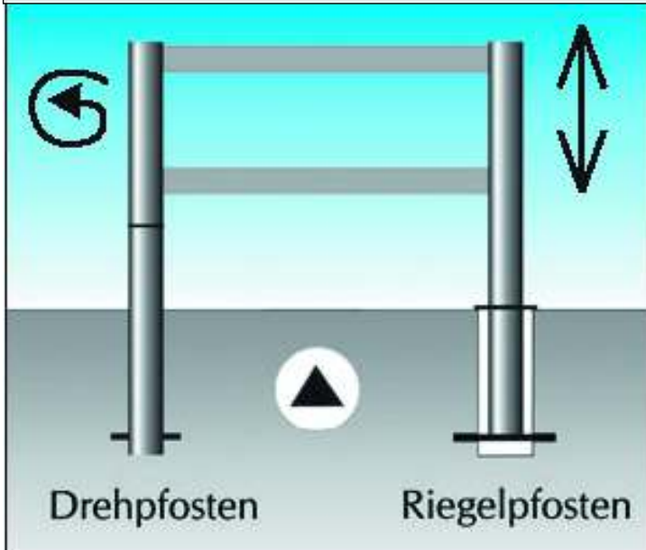
nach Entriegelung Pfosten auf einer Seite herausnehmbar
